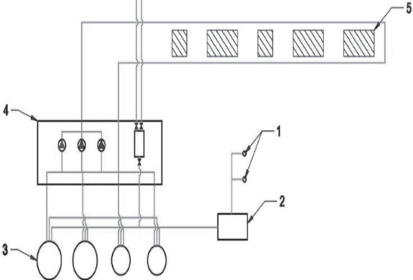
1 — водозаборные сооружения (скважины); 2 — водоочистные сооружения; 3 — резервуары чистой воды; 4 — насосы второго подъема; 5 —магистральные сети водоснабжения Рисунок 9 - Общая схема системы водоснабжения аэропорта г. Ханты-Мансийска
