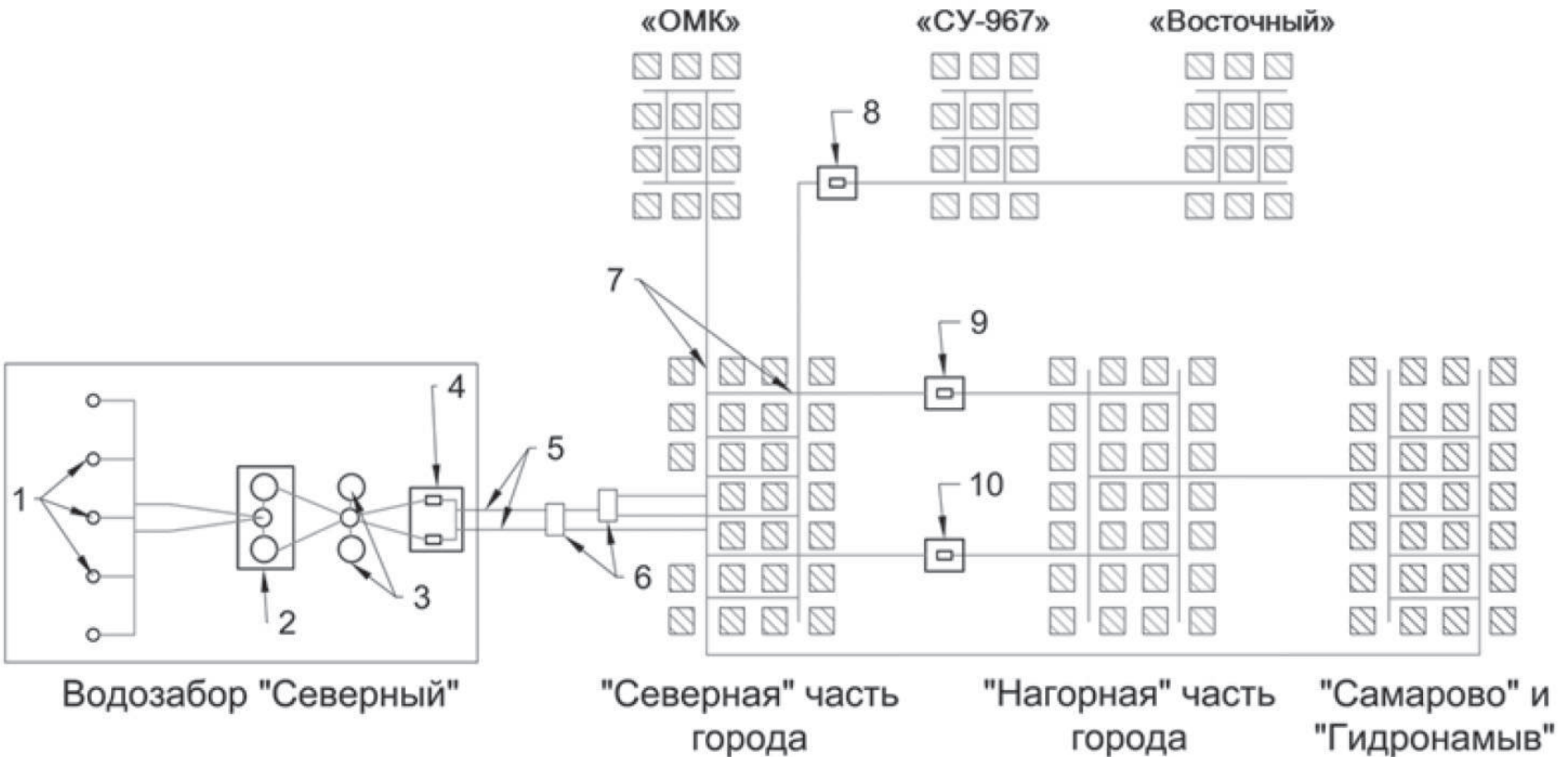
1 — водозаборные сооружения (скважины); 2 — водоочистные сооружения; 3— резервуары чистой воды; 4 — насосная станция II-го подъема; 5 — водоводы; 6 — распределительные камеры; 7—магистральные сети водоснабжения; 8— насосная станция III-го подъема «Метеостанция»; 9— насосная станция III-го подъема «Назымская»; 10 — повысительная насосная станция «Чехова д.12»; *-мкр. «Восточный» в настоящий момент находится в стадии строительства Рисунок 8 - Общая схема централизованной системы водоснабжения города Ханты-Мансийска
