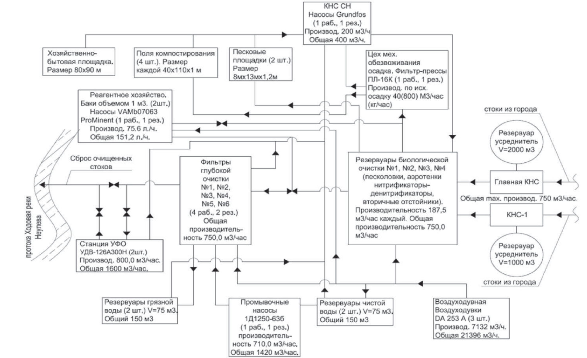
Рисунок 13 - Технологическая схема очистных сооружений бытового стока города Ханты-Мансийска, производительностью 18 000 м3/сут
